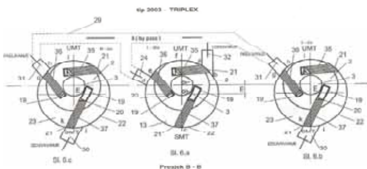
Slika 6. Šematski prikaz poprečnih presjeka cilindara, rotacionog klipa i lamela prema prijenosu br. 2.
