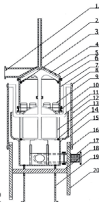
sklopni crtez br.1 poprečni presjek modifikovani izgled naprave s crteža 1. dopune pečenta
